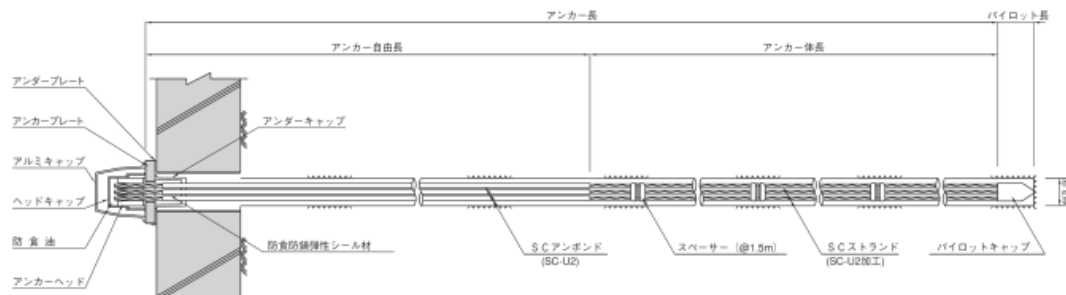
KTB・引張型SCアンカー工法の概要
