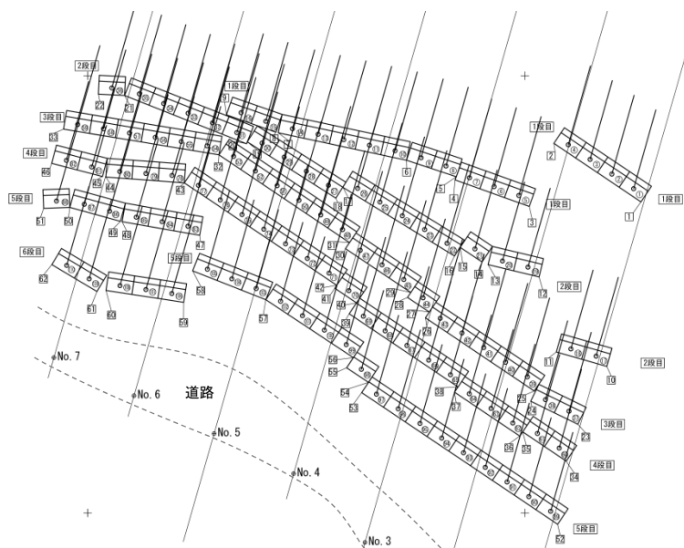
抑止工平面図
