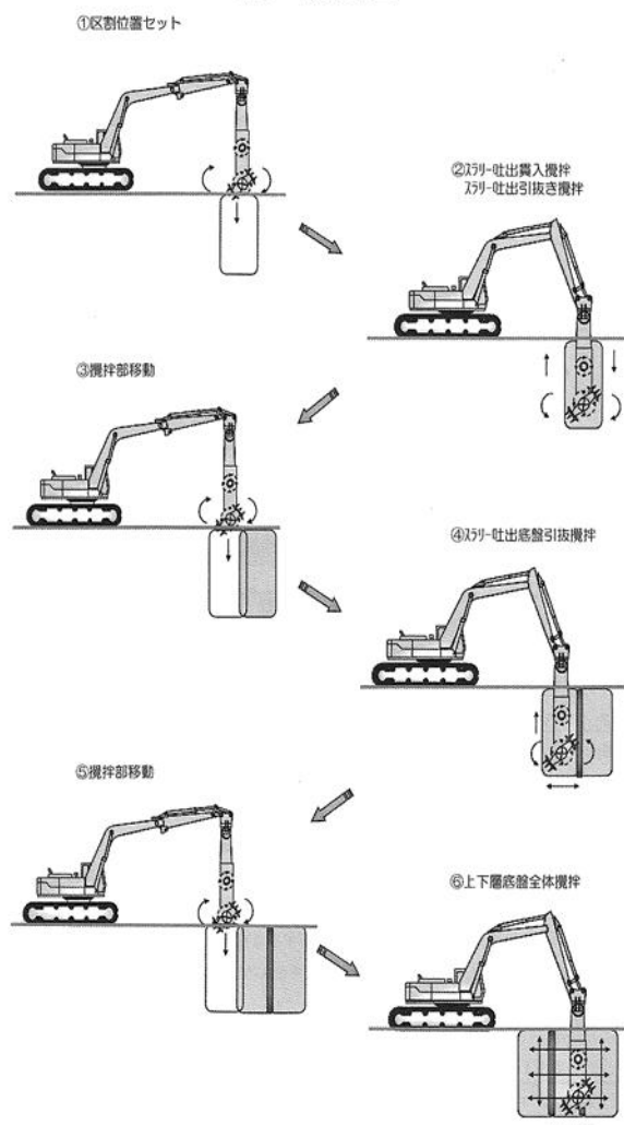
施工順序図
