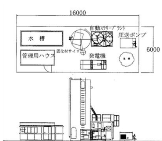
プラント配置図
