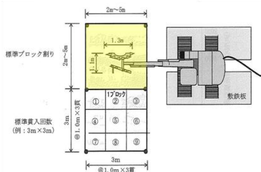
施工平面図とブロック割り図
